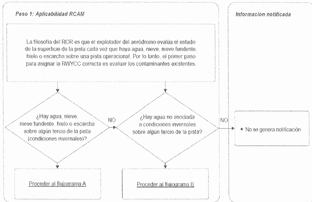
Fig. 2.5-2 El proceso básico de flujoograma de la RCAM para agua de lluvia en pista. Fuente: (figura 4-3 de la CIR 355 para las condiciones regionales)
