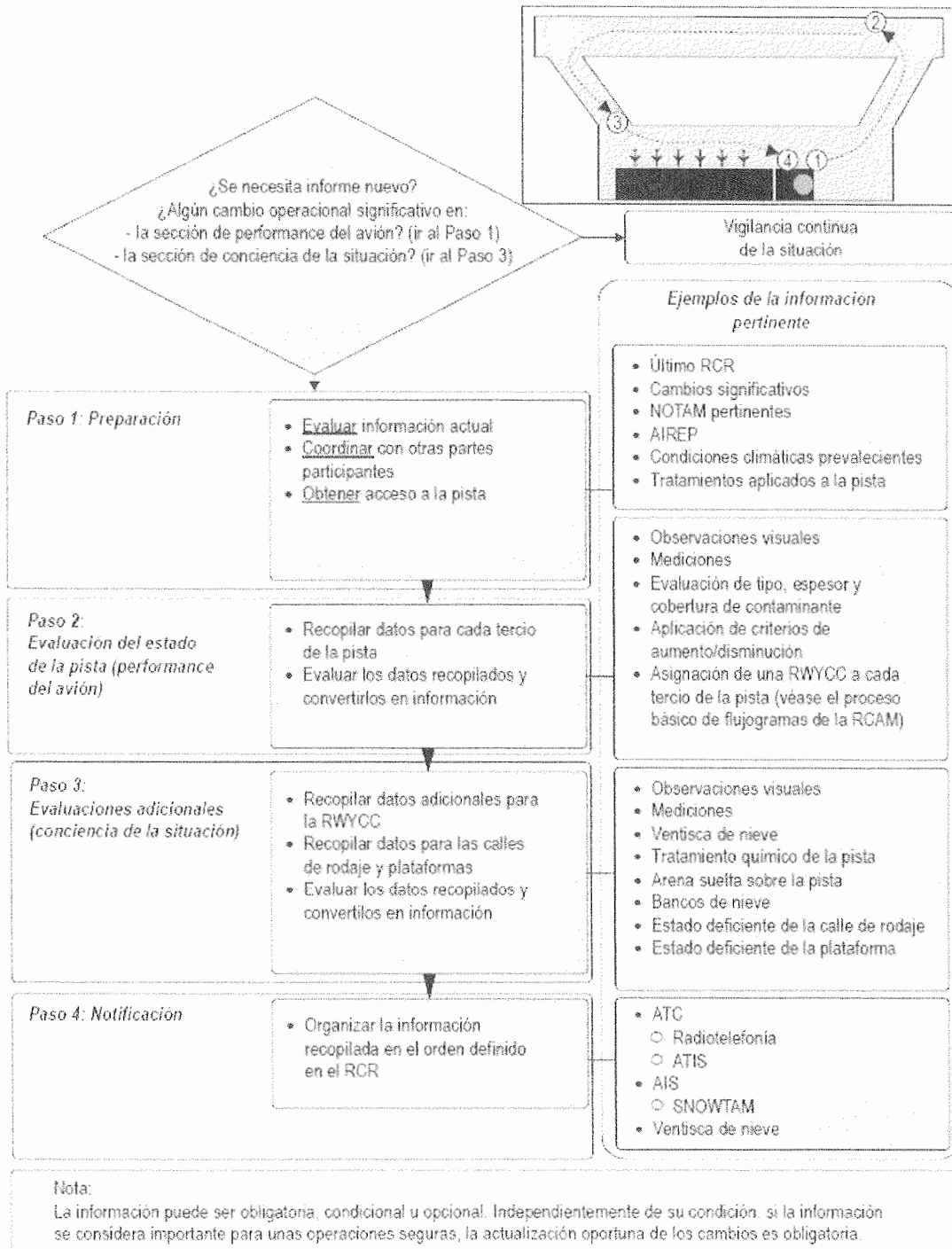
Fig. 2.5-1 Proceso genérico de evaluación del estado de la pista
