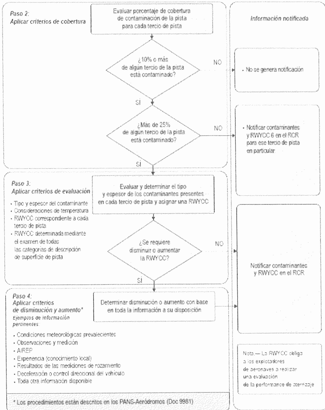
Flujograma A (Figura 4-4 de la CIR 355)
