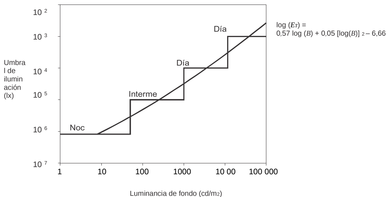
Figura D-1. Relación entre el umbral de iluminación ET (lx) y la luminancia de fondo B (cd/m 2 )
